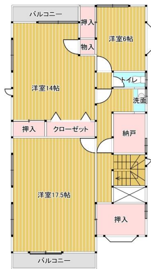
2階平面図
